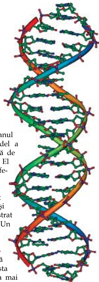
Structura moleculei de ADN care conține informația genetică a oricărei celule
