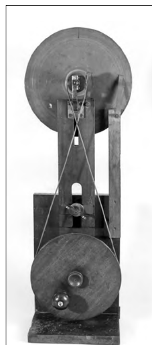
Discul lui Faraday – 1831. Primul generator electric.
