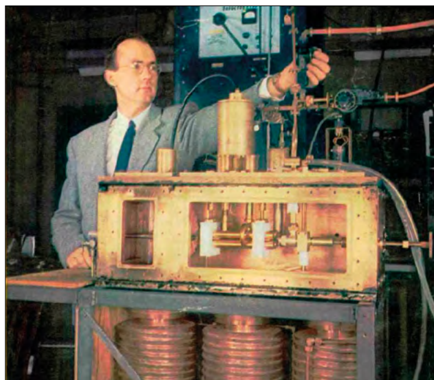
Charles H. Townes și primul maser (1955), precursorul laser-ului.
